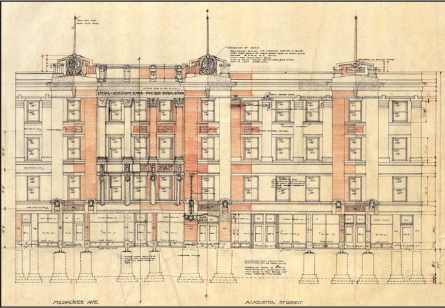
Plan fasady budynku biura głównego ZPRKA wg. architekta p. J. Flizikowskiego
